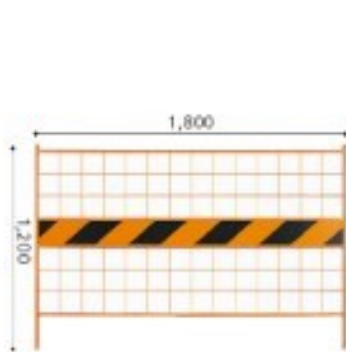
地域仕様 中型上下網フェンス 九州 標準仕様 商品コード 1632 外形サイズ 縦1,200×横1,800mm
