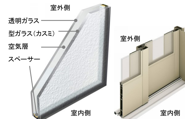
※複層ガラス入完成品のガラスは、室内側の空気層面が型ガラス(カスミ)になっています。
