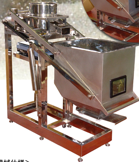
【原料投入時】
