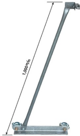
アングルベース 控金具 L=1,000mm 単重:1.8kg
