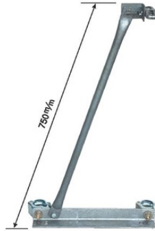
ミニフェンス用 アングルベース控金具 L=750mm 単重:1.48kg
