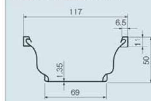
軒どい(117)断面図 (位単:mm)
