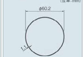
たてどい(60)断面図
