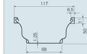
軒どい(117)断面図(位単:mm)
