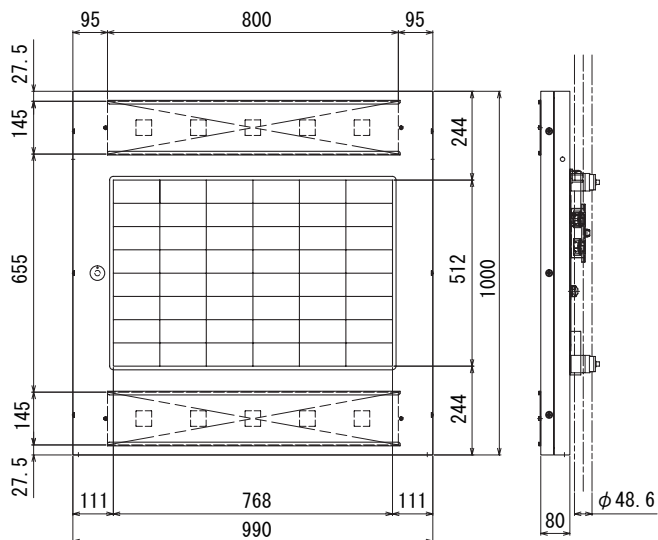
■寸法図
