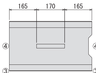
■下部平面図
