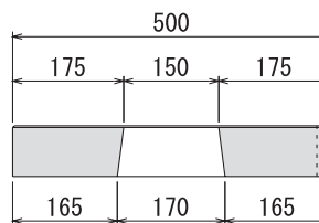
■④—④断面図
