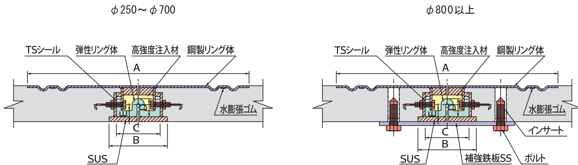
■ 可とう部概要図
