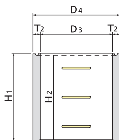
■直壁
