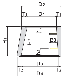
■斜壁
