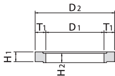
■調整リング
