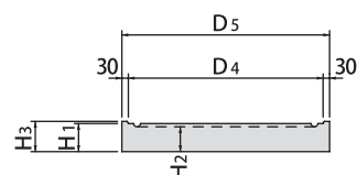
■底板
