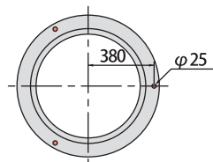
■直壁
