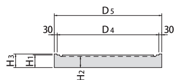
■底板
