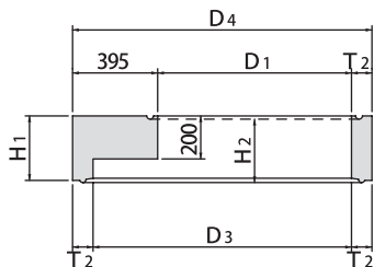
■床版
