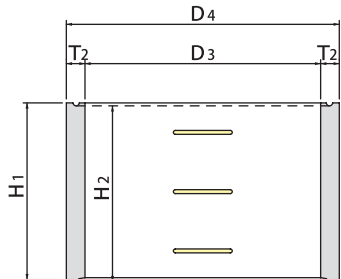
■直壁
