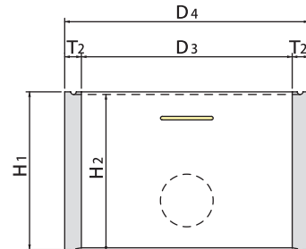
■管取付壁
