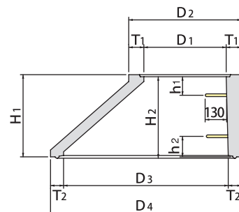
■斜壁
