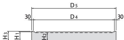
■底板
