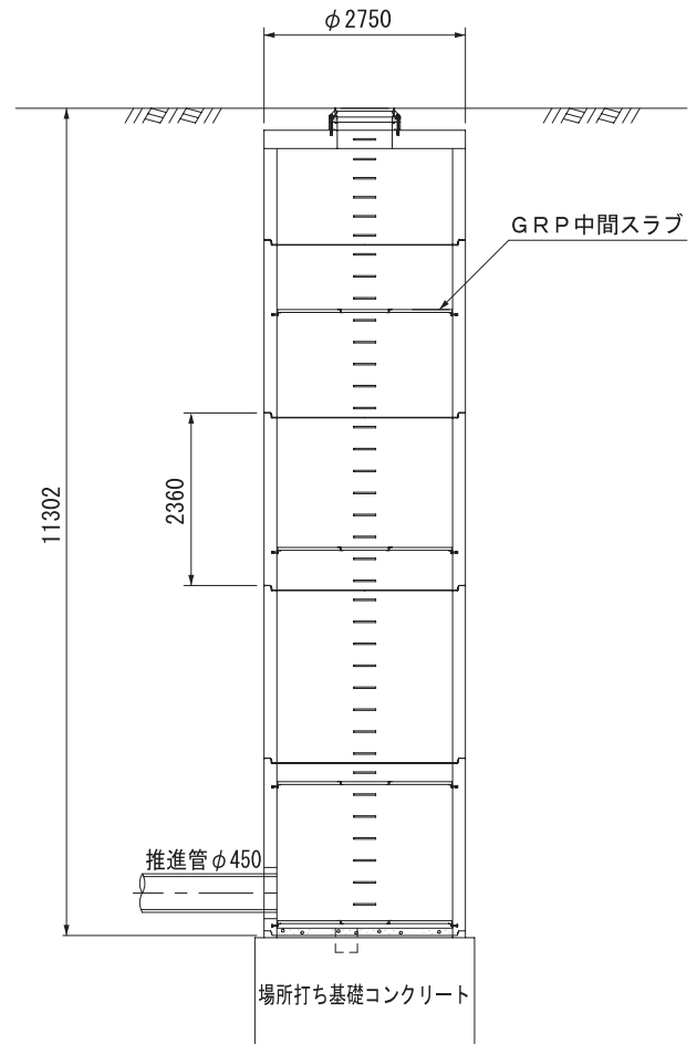
■横断面図
