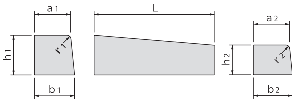
大中寸法図
