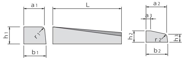
小寸法図
