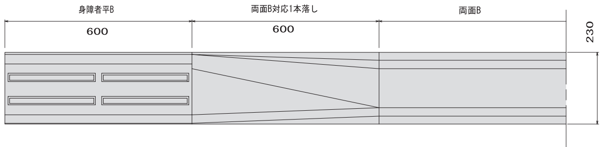
■側面図
