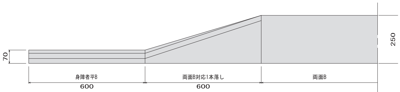
■側面図
