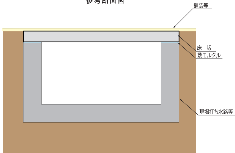
参考断面図
