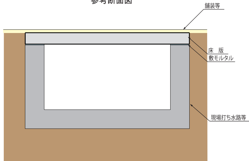
参考断面図
