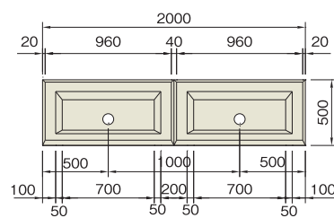
正面図
