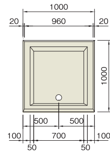
正面図
