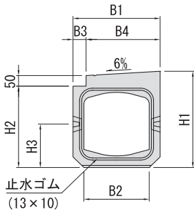
■内部断面図
