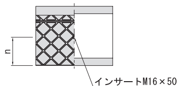
■平面図
