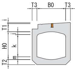
■内部断面図
