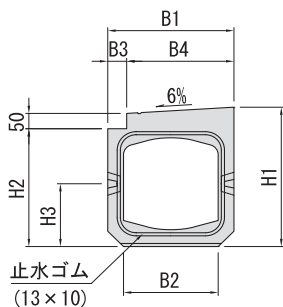
■内部断面図
