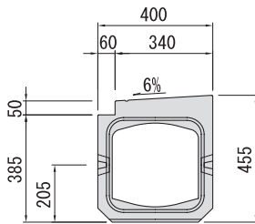
■ 端部正面図
