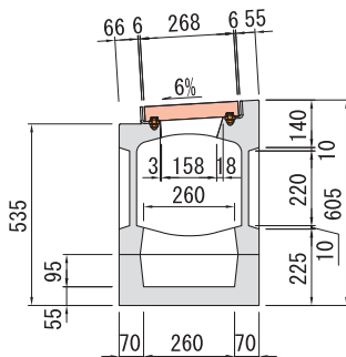
■ 中央断面図
