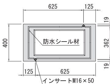
■ 柵部上面図
