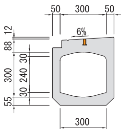
■ 端部断面図
