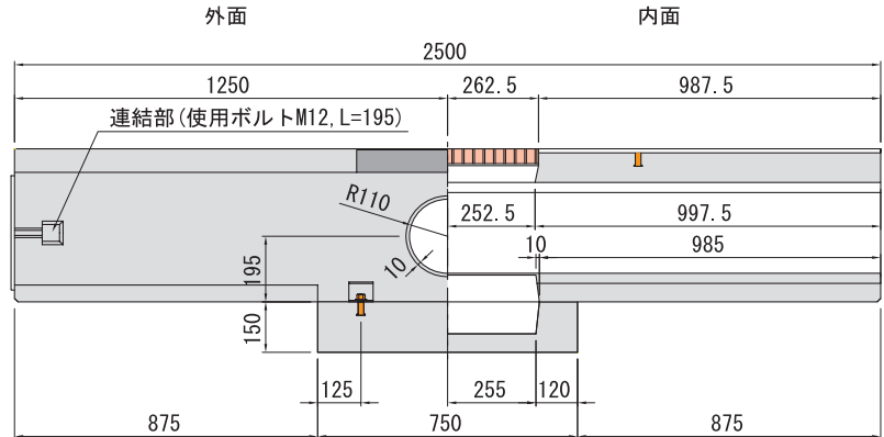
■ 側面図
