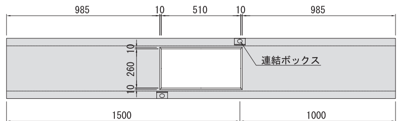
■ 底部平面図
