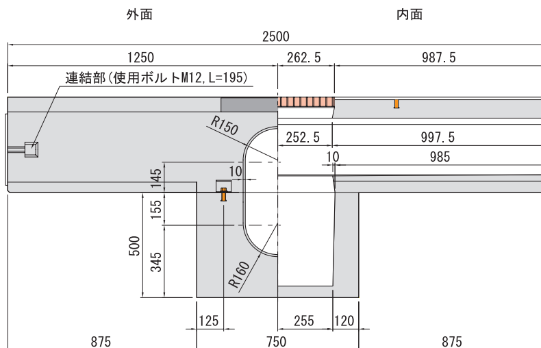
■側面図
