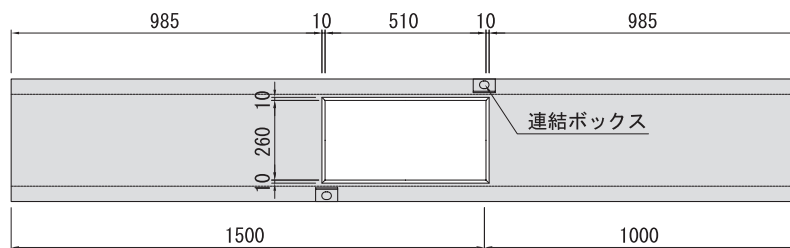
■底部平面図
