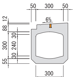
■端部断面図
