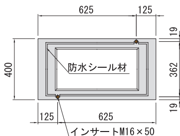
■柵部上面図
