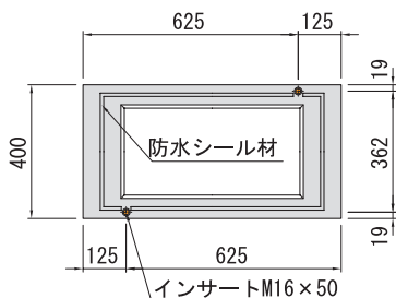
■枡部上面図
