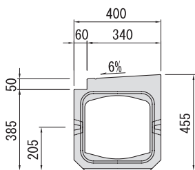
■端部正面図
