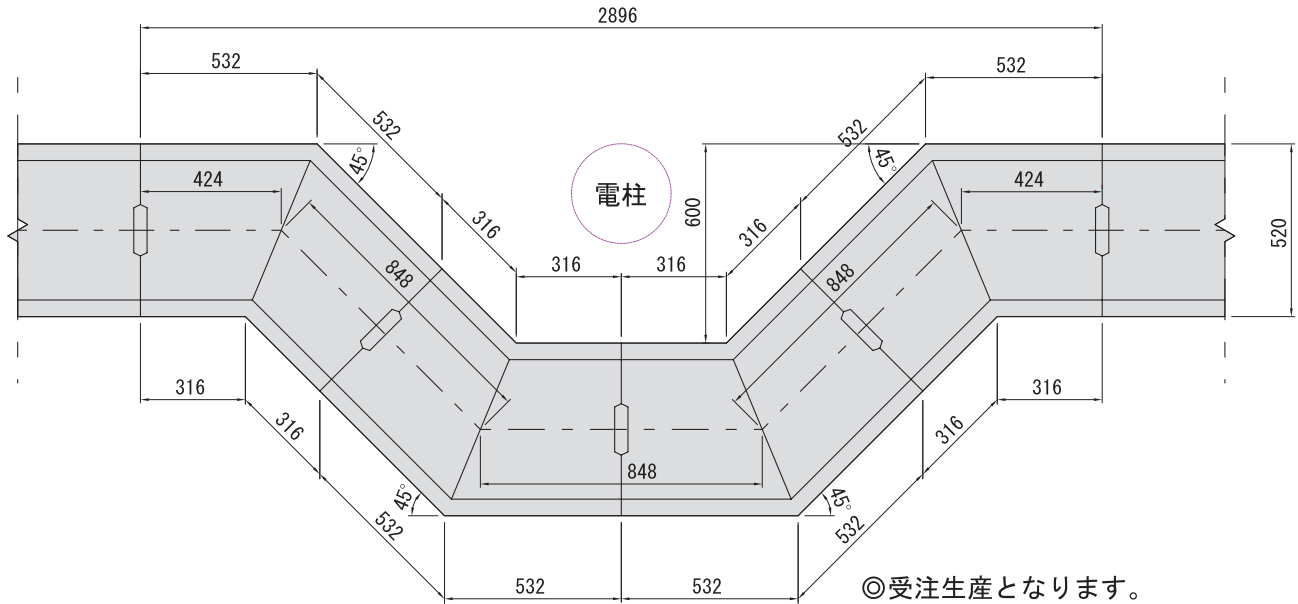
■蓋部平面図
