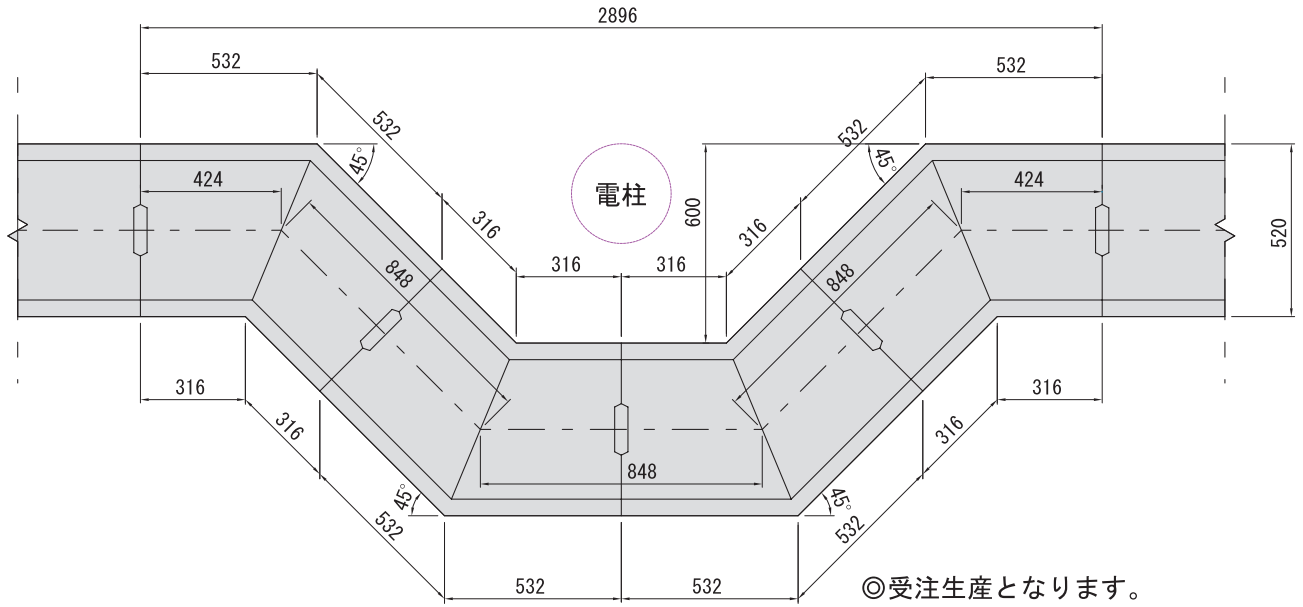
■蓋部平面図
