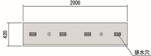
CCタイプ (横断-暗渠)
