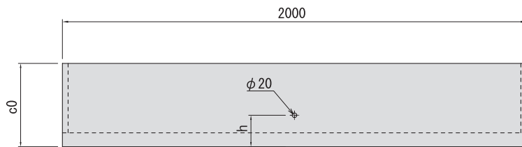
■側面図
