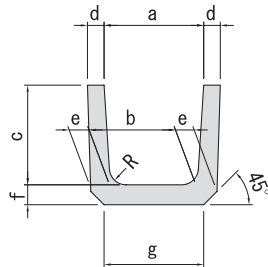
■断面図
