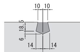
■モルタル目地溝詳細図
