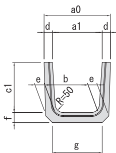
■断面図
