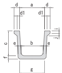
■差し口断面図
