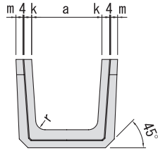
■受け口断面図
