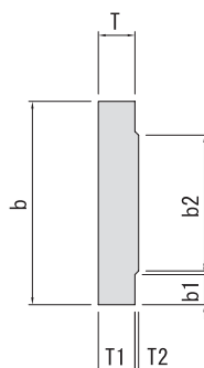
■側面図
