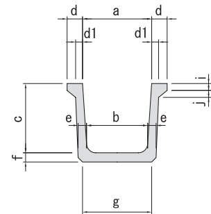
■差し口断面図
