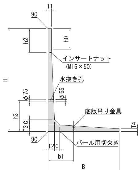
■断面図
