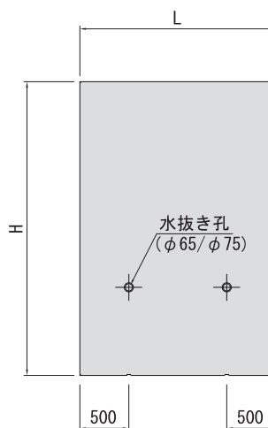
■正面図
