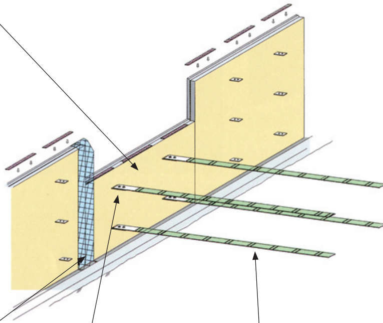
【厚み 140 フルサイズ（約 1100kg）】
