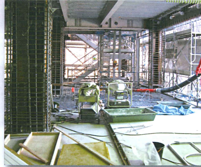
4. 炭素繊維補強工事例
