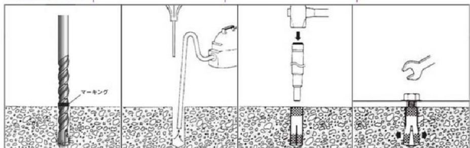
① 所定の径・深さに穿孔。
