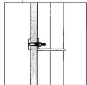
ダクト吊り金具取り付け
