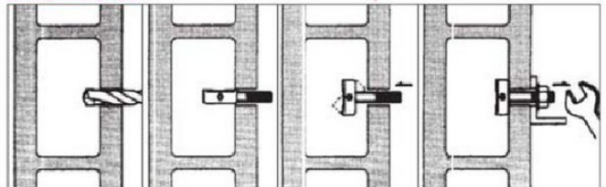
①所定の径で穿孔。②アマラハンガーを挿入。③ロールプレート部が中空部に出ると自然に落ちる。④ナットを締め付け、施工完了。
