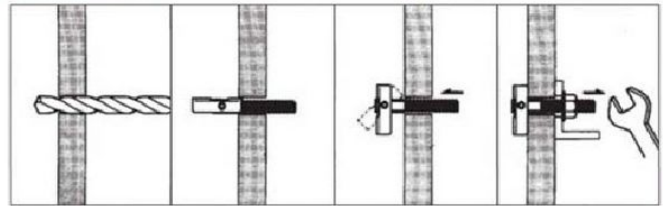
①所定の径で穿孔。②ITハンガーを挿入。③ロールプレート部が中空部に出ると自然に落ちる。④ナットを締め付け、施工完了。
