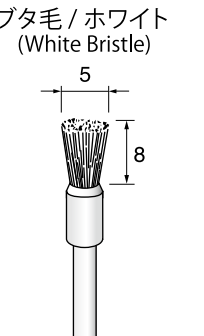
軸径φ3.0mm (φ3.0 shank φ3.0軸直径)
