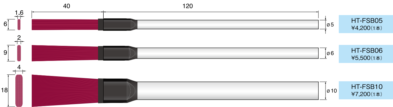
1 ファイバーストーンハンドブラシ Fiber Stone Hand Brush #1200相当 線径 ■ 約0.3mm
