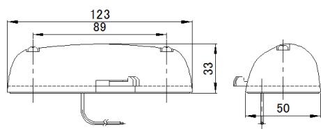
NM3 24V80W シールドビーム単体
