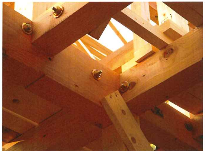
タイトニック耐震座金
