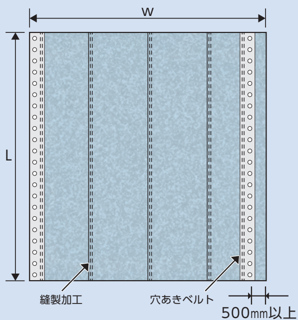
標準加工図
