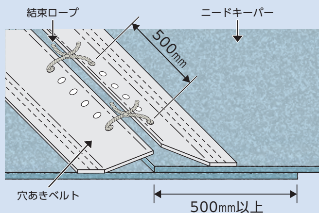
重ね継手部詳細図
