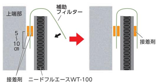
補助フィルター参考取付図
