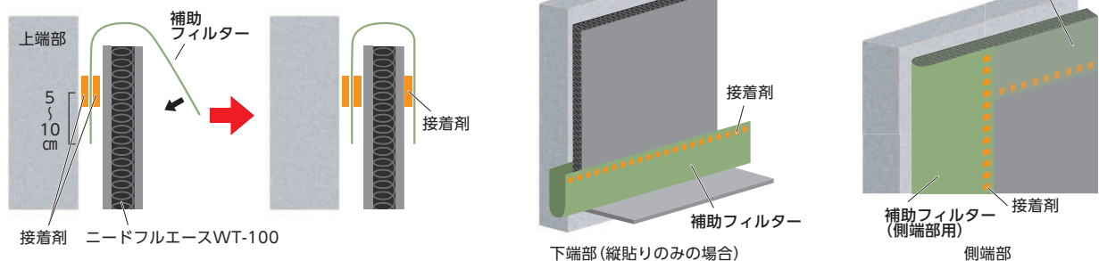
補助フィルター参考取付図
