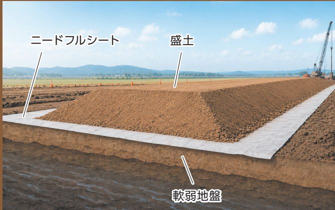
軟弱地盤土地改良工法
