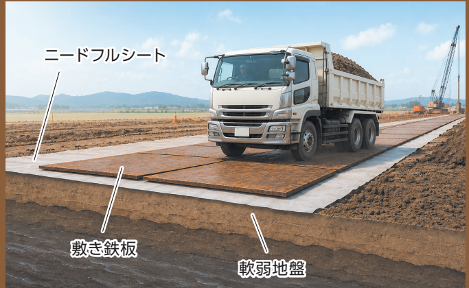
軟弱地盤でのトラフィカビリティの確保
