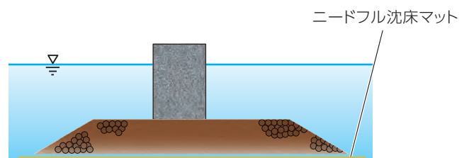
防波堤等の洗掘防止工
