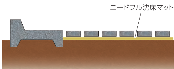
河川護床工
