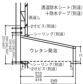
■標準納まり
