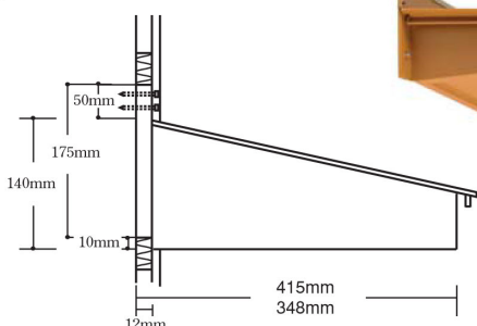
■標準納まり
