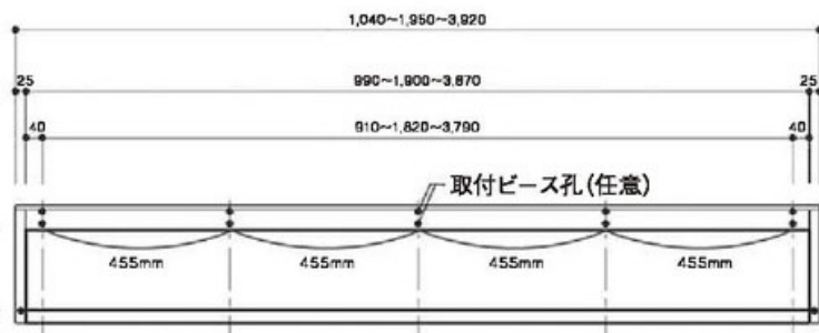
正面図
