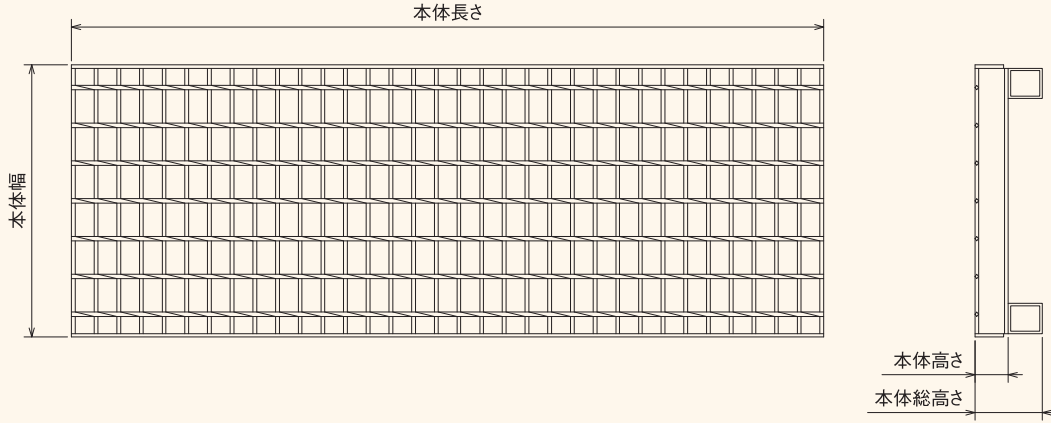
本図は溝幅250用のMタイプを表示しています
