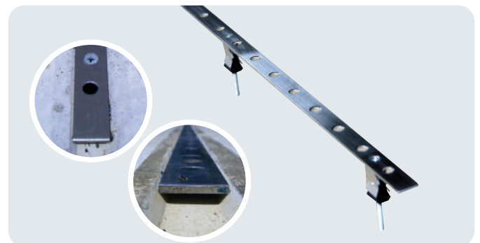
スリット側溝蓋 ズレ止め／跳上防止機能付(特許申請中)
