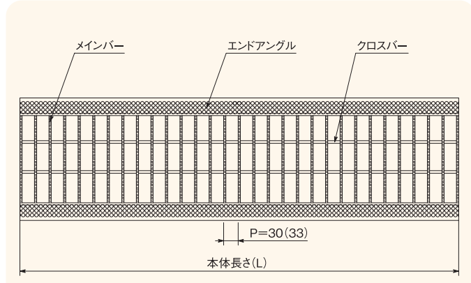
本図は溝幅300用を表示しています
