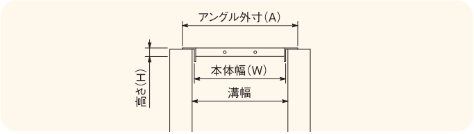
本図は溝幅300用を表示しています
