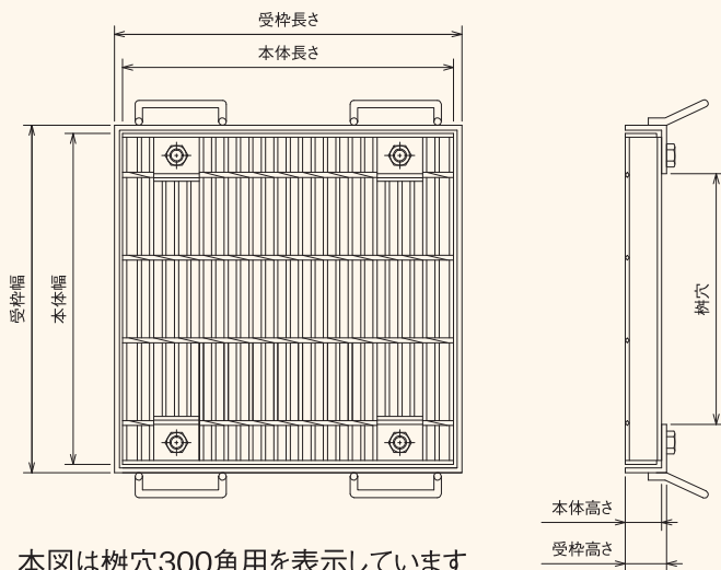
本図は樹穴300角用を表示しています
