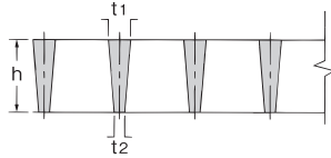
▼ 断面図
