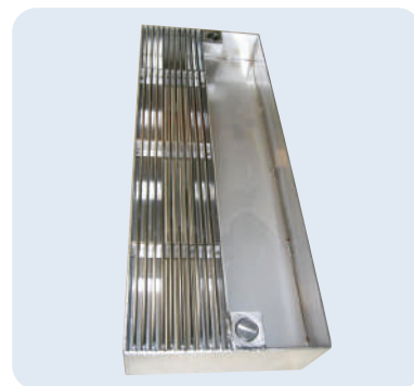
スリット(特殊タイプ) 集水枳
