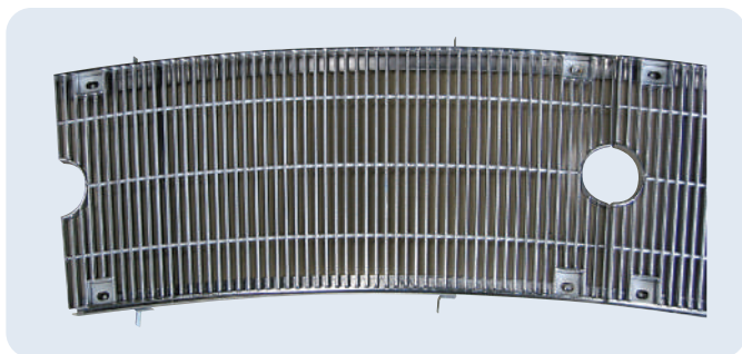
R加工／ボルト固定式グレーチング
