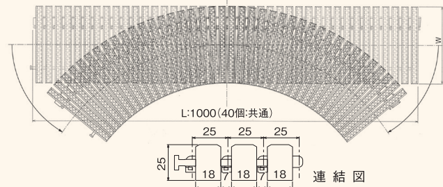
RG-R／曲線タイプ連結図(1m)
