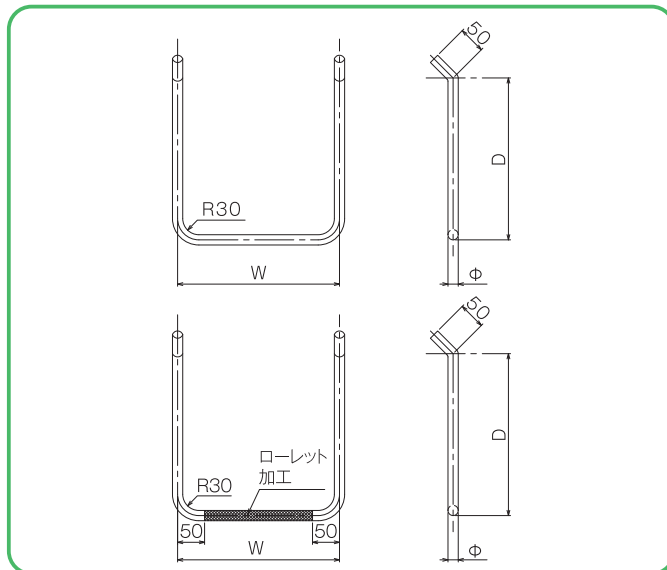
YRT〈ローレットタイプ〉 ●型式記号・仕様・重量・価格表
